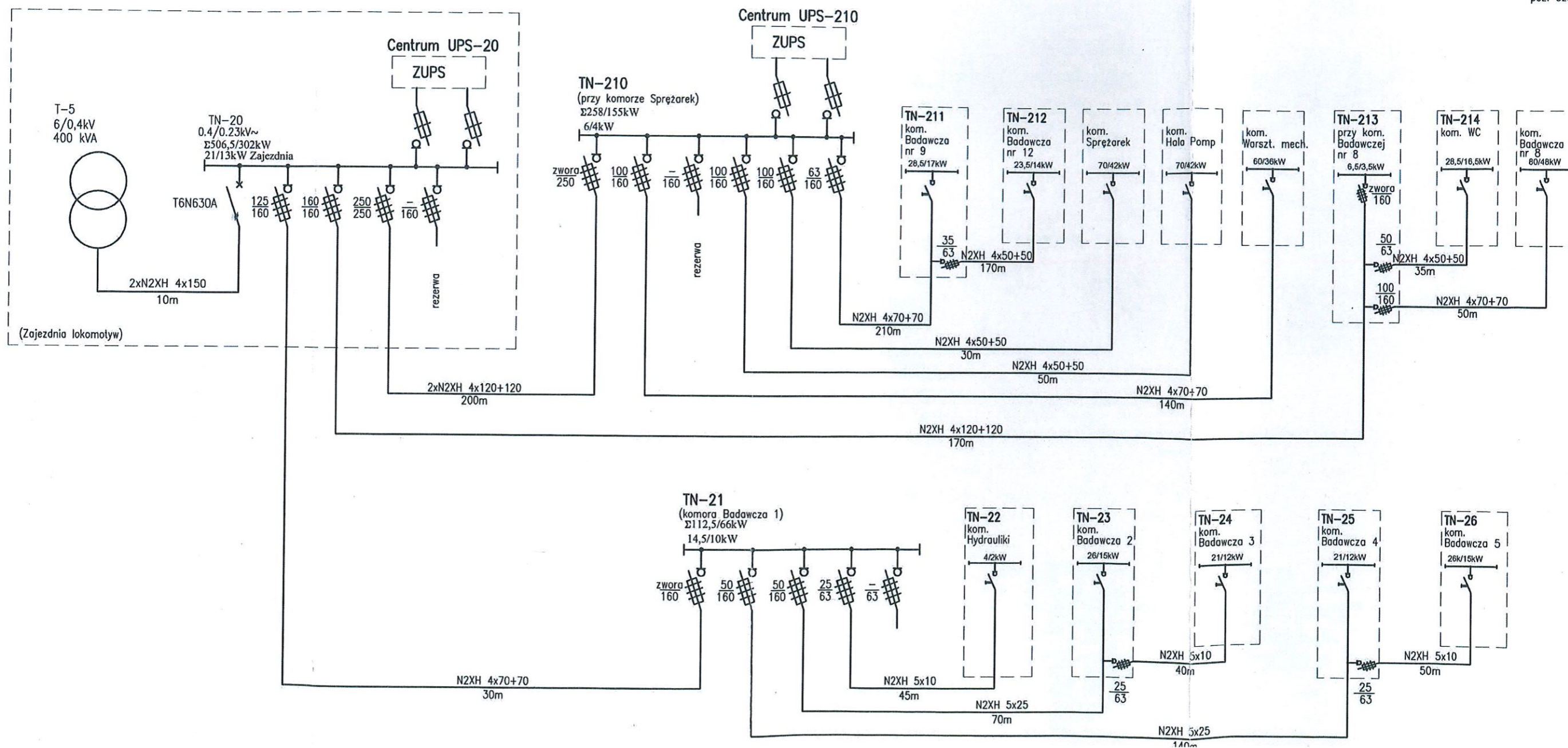
Tytuł rysunku: Schemat strukturalny sieci 400/230V na poz. 320
