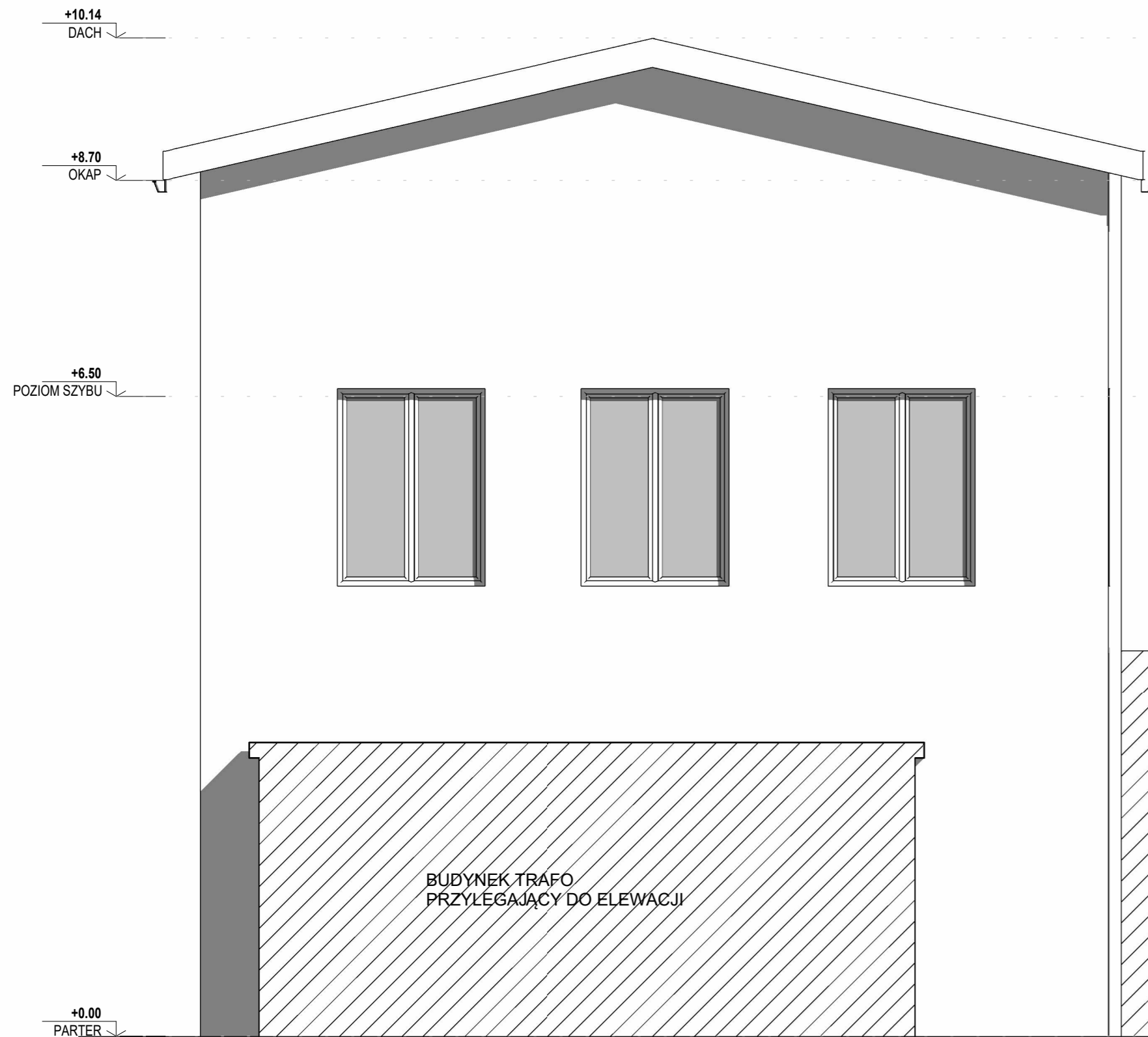
1 ELEWACJA WSCHODNIA 1 : 50
